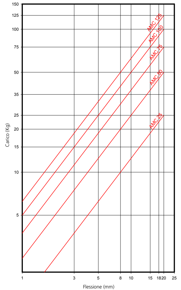
AMC CARICO DEFORMAZIONE MECANOCAUCHO® Tipo Serie media
