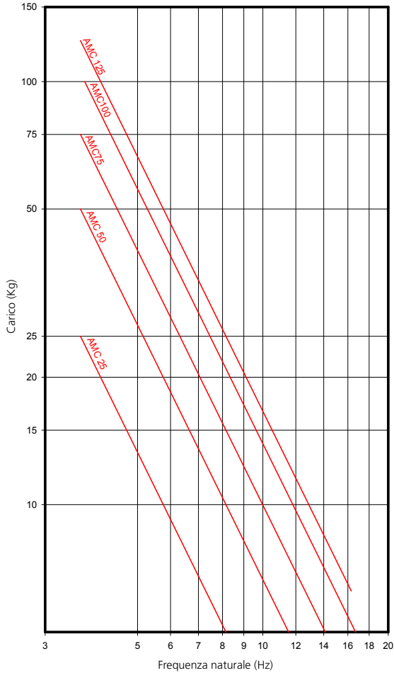
AMC FREQUENZE PROPRIE MECANOCAUCHO® Tipo Serie media
