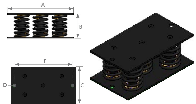
AMC CARICO DEFORMAZIONE MECANOCAUCHO® Tipo 5 AMC
