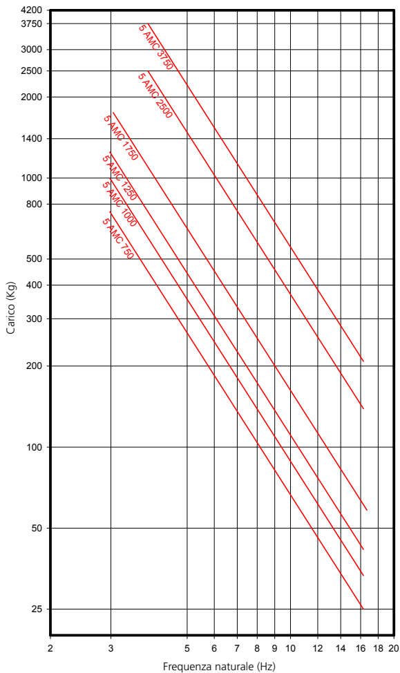
AMC FREQUENZE PROPRIE MECANOCAUCHO® Tipo 5 AMC
