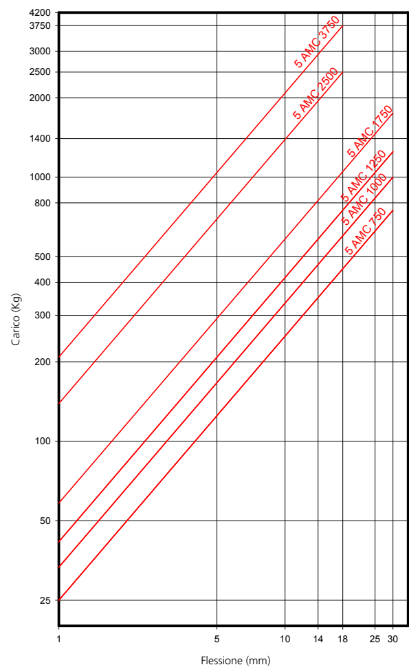
AMC CARICO DEFORMAZIONE MECANOCAUCHO® Tipo 5 AMC
