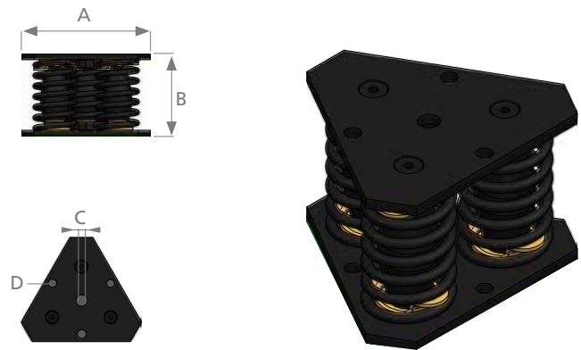
AMC CARICO DEFORMAZIONE MECANOCAUCHO® Tipo 3 AMC
