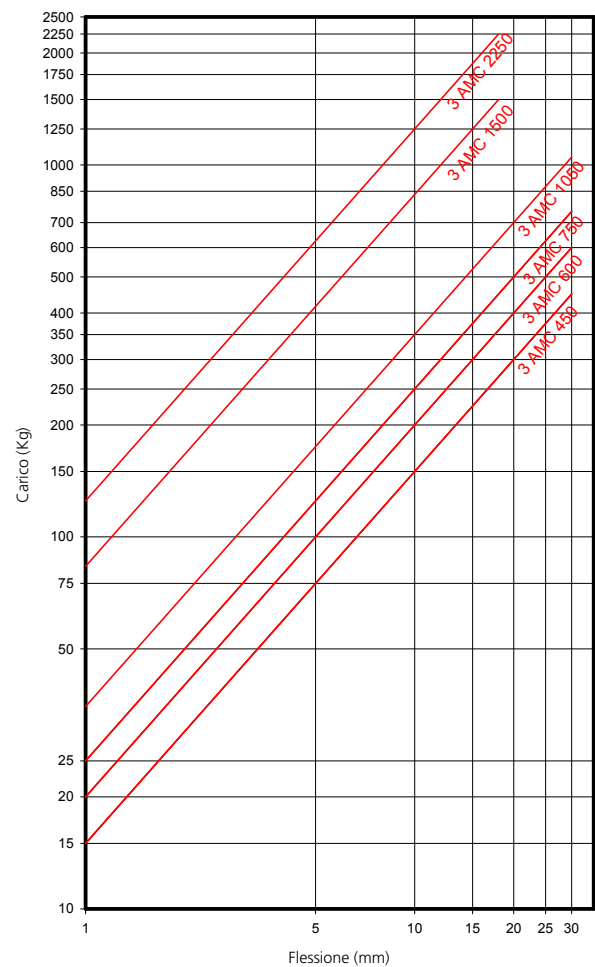
AMC CARICO DEFORMAZIONE MECANOCAUCHO® Tipo 3 AMC
