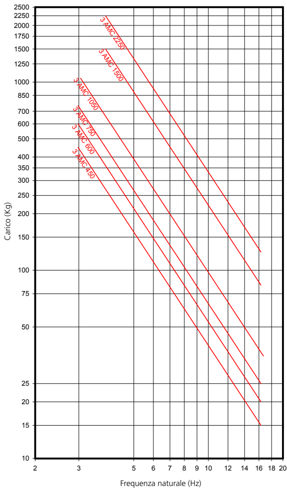
AMC FREQUENZE PROPRIE MECANOCAUCHO® Tipo 3 AMC
