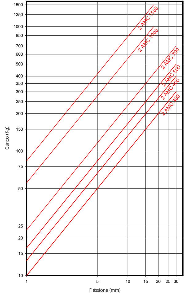
AMC CARICO DEFORMAZIONE MECANOCAUCHO® Tipo 2 AMC
