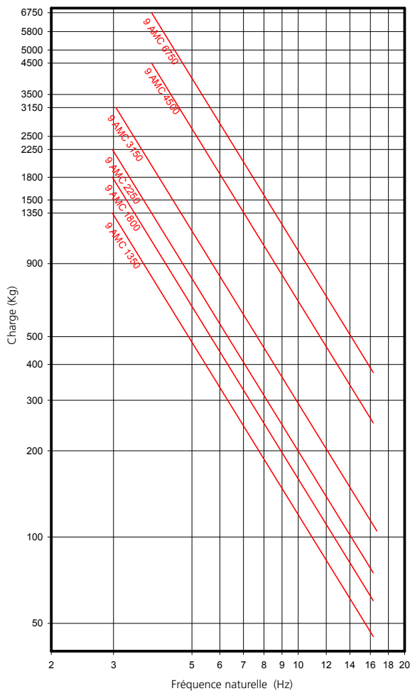
AMC FRÉQUENCES PROPRES MECANOCAUCHO® Type 9 AMC
