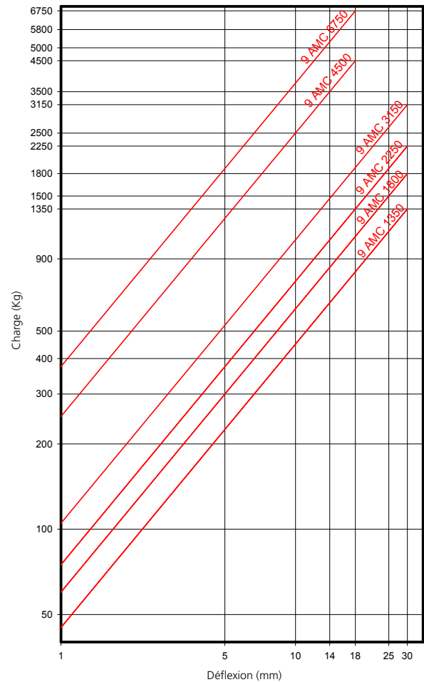
AMC CHARGE DÉFORMATION MECANOCAUCHO® Type 9 AMC
