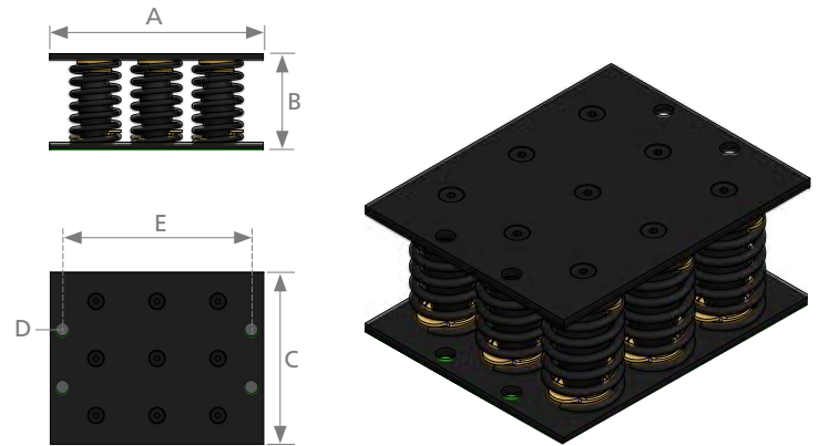
AMC CHARGE DÉFORMATION MECANOCAUCHO® Type 9 AMC
