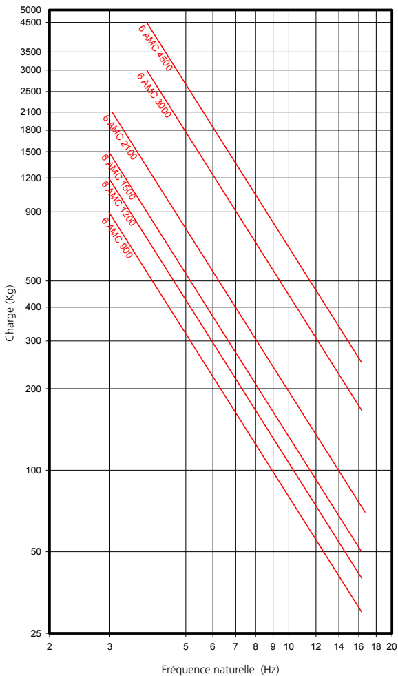
AMC FRÉQUENCES PROPRES MECANOCAUCHO® Type 6 AMC
