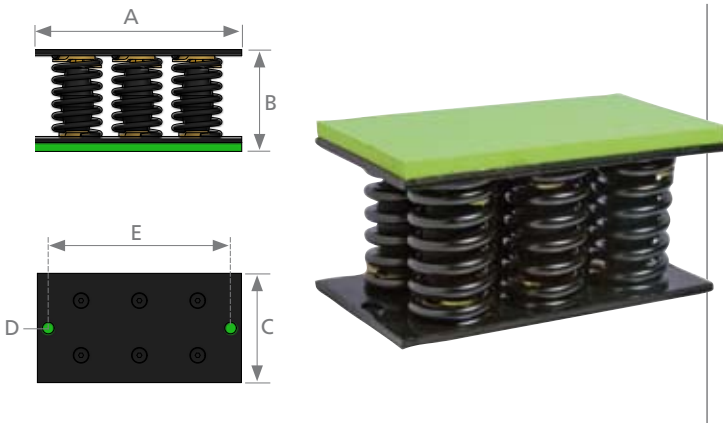
AMC FRÉQUENCES PROPRES MECANOCAUCHO® Type 6 AMC
