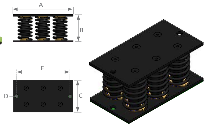
AMC CHARGE DÉFORMATION MECANOCAUCHO® Type 6 AMC
