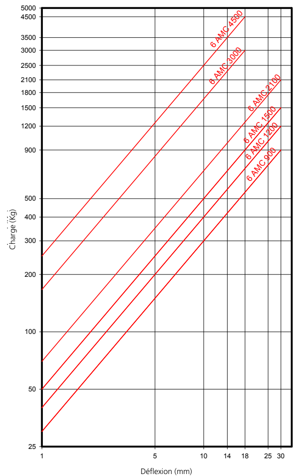
AMC CHARGE DÉFORMATION MECANOCAUCHO® Type 6 AMC
