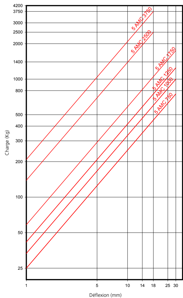
AMC CHARGE DÉFORMATION MECANOCAUCHO® Type 5 AMC
