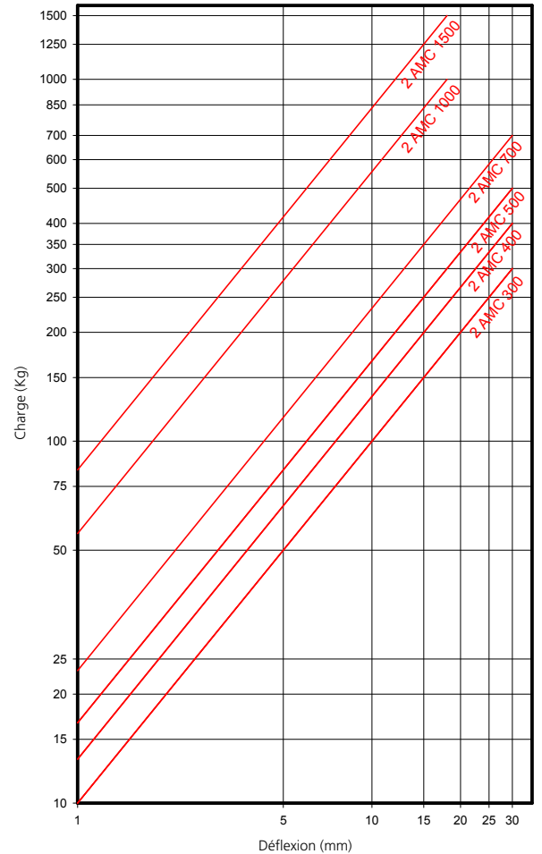
AMC CHARGE DÉFORMATION MECANOCAUCHO® Type 2 AMC
