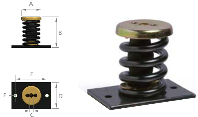
AMC CHARGE DÉFORMATION MECANOCAUCHO® Type 1 AMC
