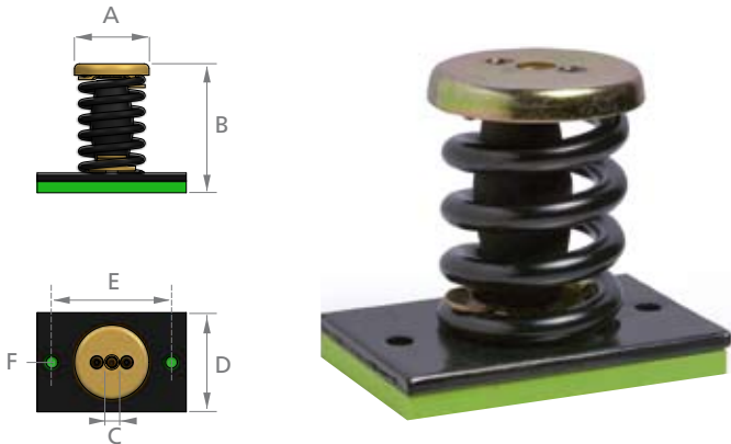
AMC FRÉQUENCES PROPRES MECANOCAUCHO® Type 1 AMC
