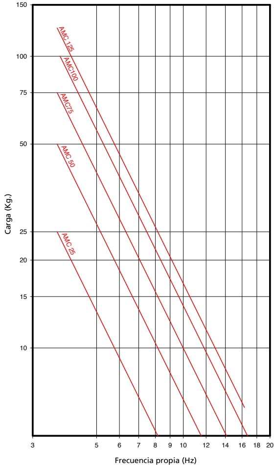
AMC FRECUENCIAS PROPIAS MECANOCAUCHO® Tipo Serie media
