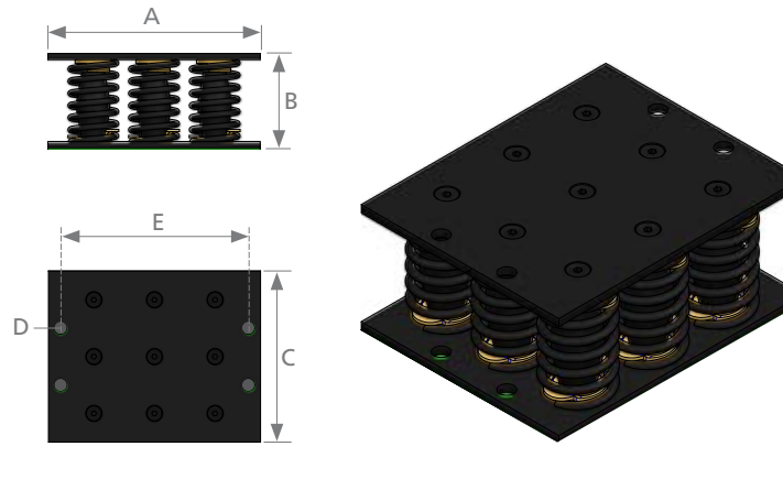
AMC CARGA DEFORMACION MECANOCAUCHO® Tipo 9 AMC
