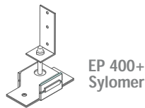
EP+ Sylomer Tipo A
