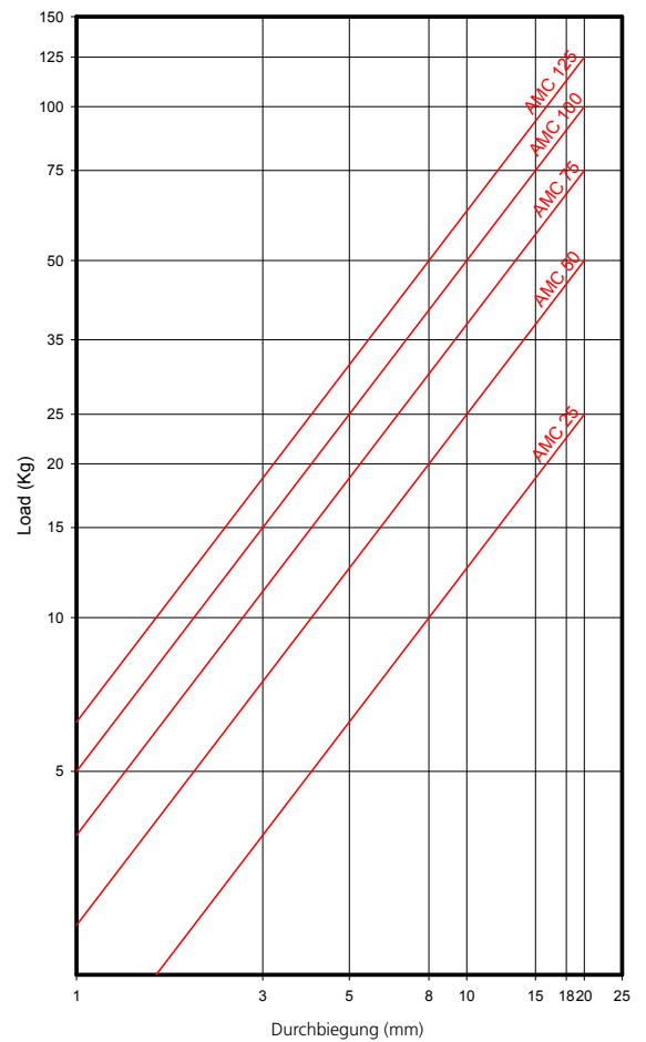
AMC BELASTUNGSDEFORMATION MECANOCAUCHO Typ mittlere Serie
