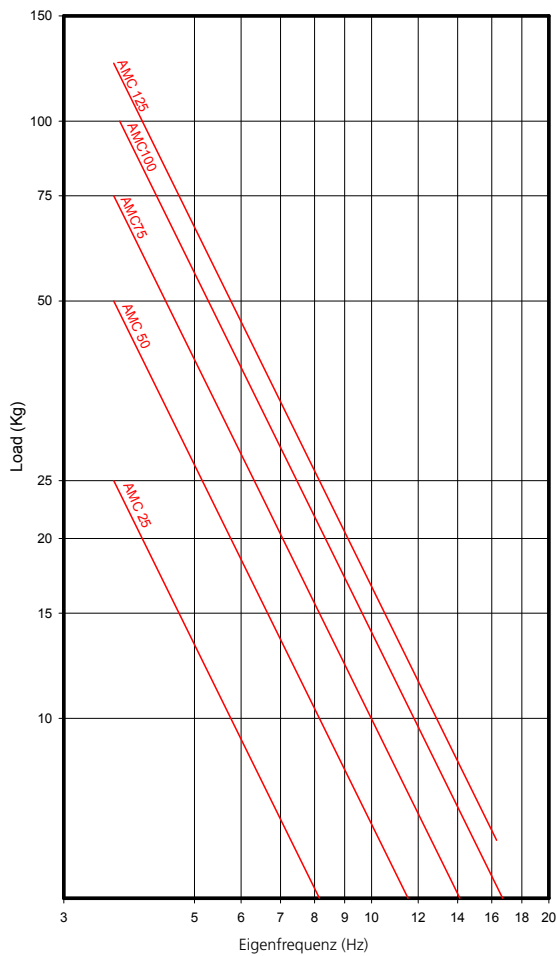
AMC EIGENFREQUENZEN MECANOCAUCHO Typ mittlere Serie
