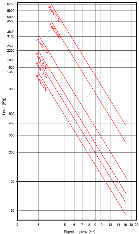
AMC EIGENFREQUENZEN MECANOCAUCHO TYP 9 AMC
