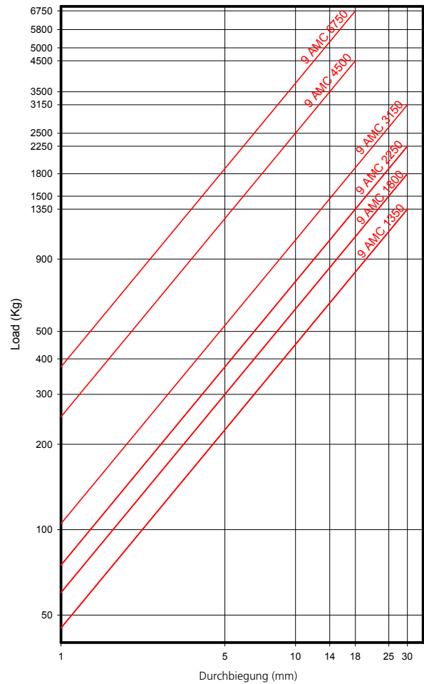
AMC BELASTUNGSDEFORMATION MECANOCAUCHO TYP 9 AMC
