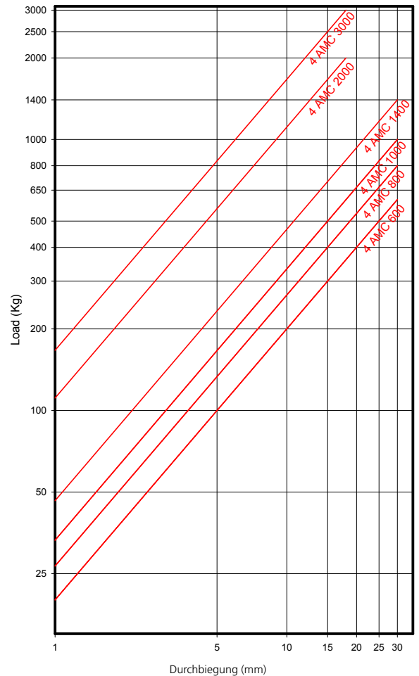
AMC BELASTUNGSDEFORMATION MECANOCAUCHO TYP 4 AMC
