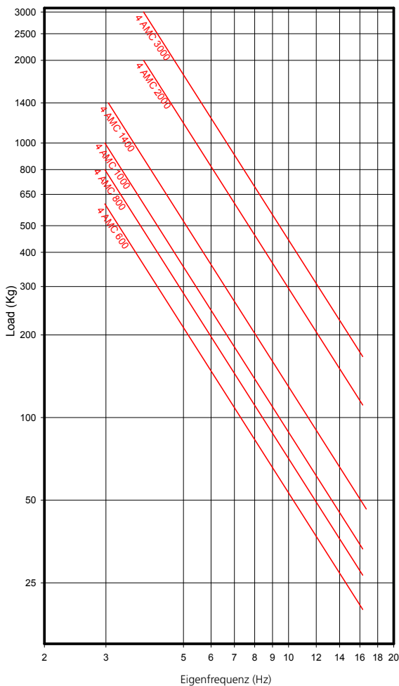
AMC EIGENFREQUENZEN MECANOCAUCHO TYP 4 AMC
