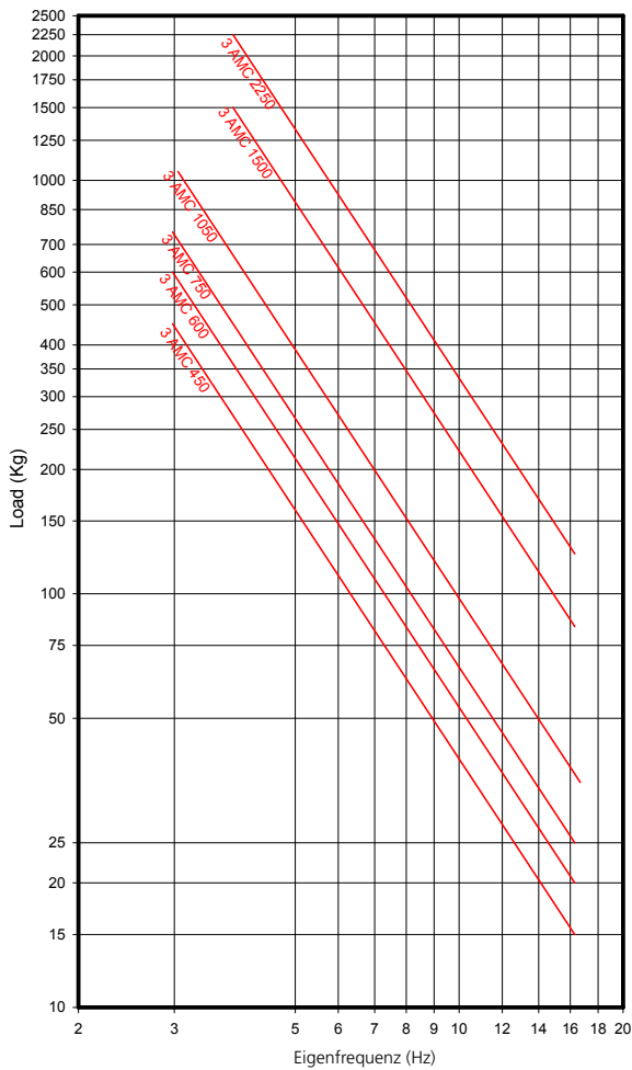
AMC EIGENFREQUENZEN MECANOCAUCHO TYP 3 AMC
