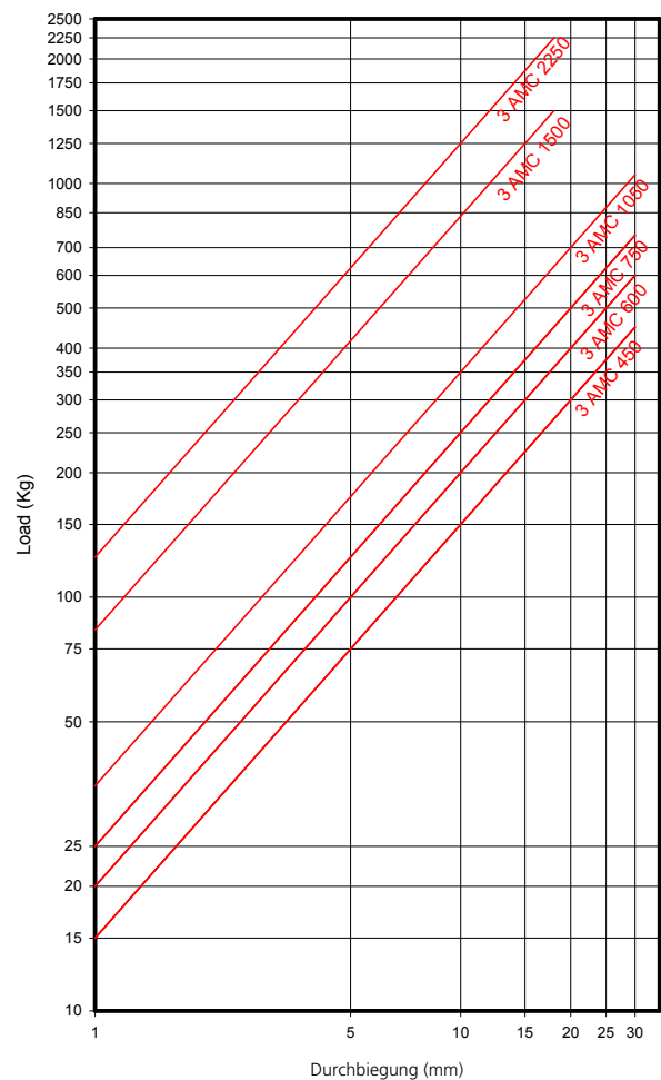
AMC BELASTUNGSDEFORMATION MECANOCAUCHO TYP 3 AMC
