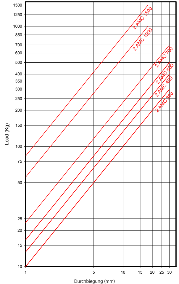
AMC BELASTUNGSDEFORMATION MECANOCAUCHO TYP 2 AMC
