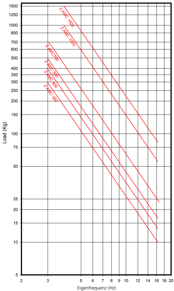
AMC EIGENFREQUENZEN MECANOCAUCHO TYP 2 AMC
