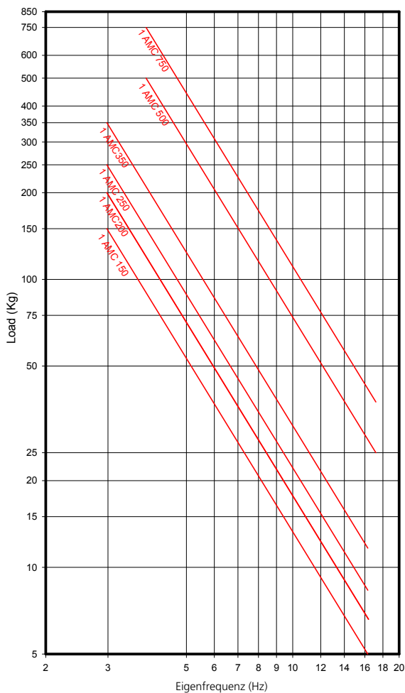
AMC EIGENFREQUENZEN MECANOCAUCHO TYP 1 AMC
