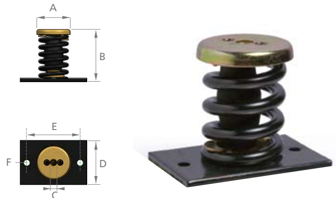
AMC BELASTUNGSDEFORMATION MECANOCAUCHO TYP 1 AMC
