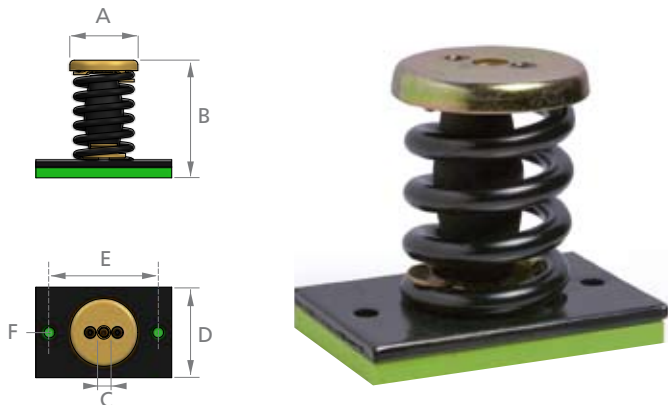
AMC EIGENFREQUENZEN MECANOCAUCHO TYP 1 AMC
