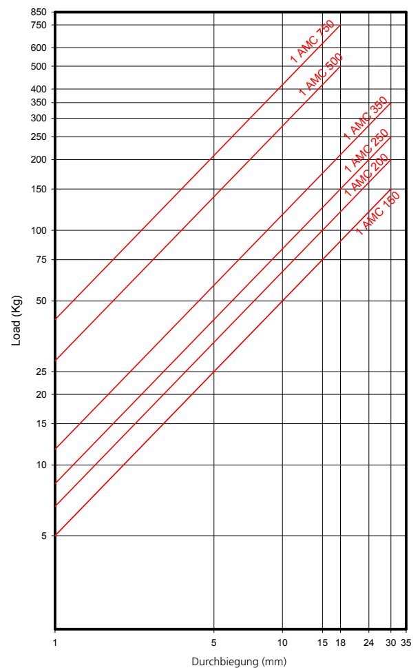
AMC BELASTUNGSDEFORMATION MECANOCAUCHO TYP 1 AMC
